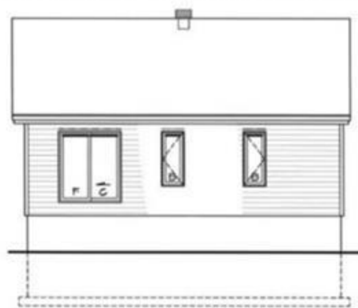
ELEV. ARRIERE
