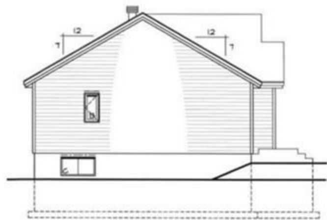
ELEV. GAUCHE
