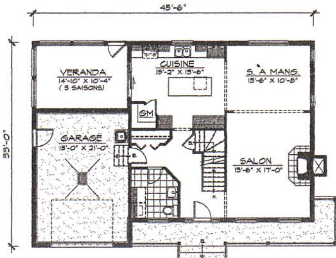
REZ-DE-CHAUSSÉE
