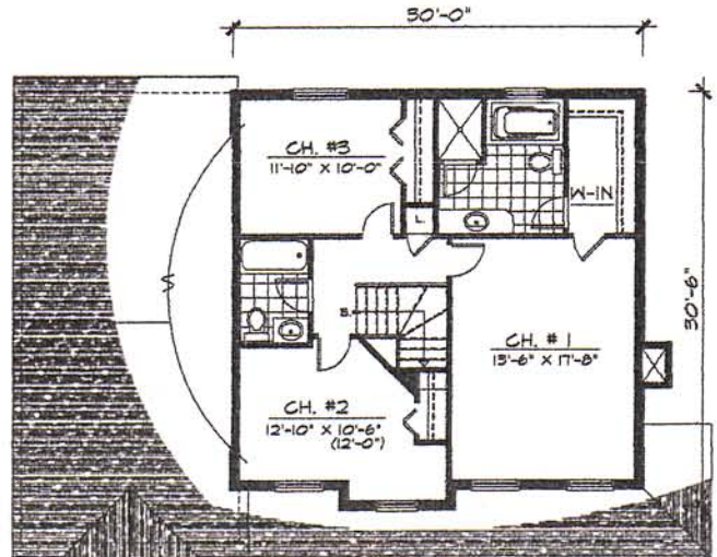
ÉTAGE
